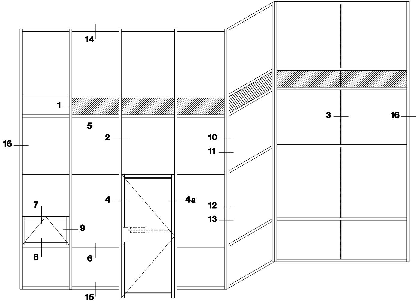
ELEVATION
